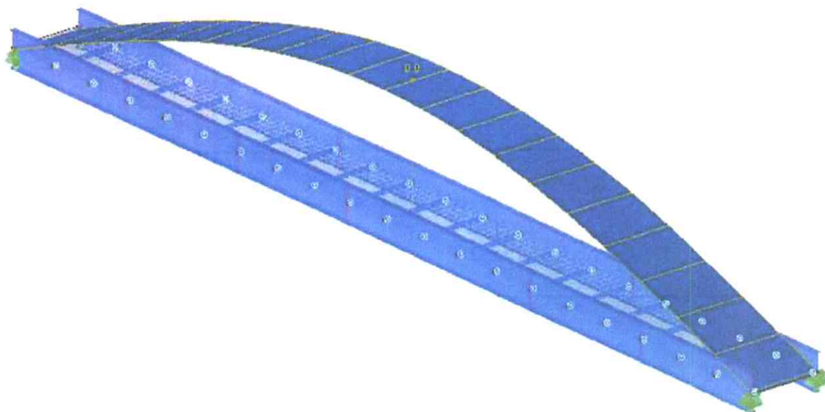
Obr. 4.4 – I. vlastní tvar nezatížené konstrukce, ztužené monolitickou spřaženou betonovou deskou, f_1 = 2,06 Hz.
