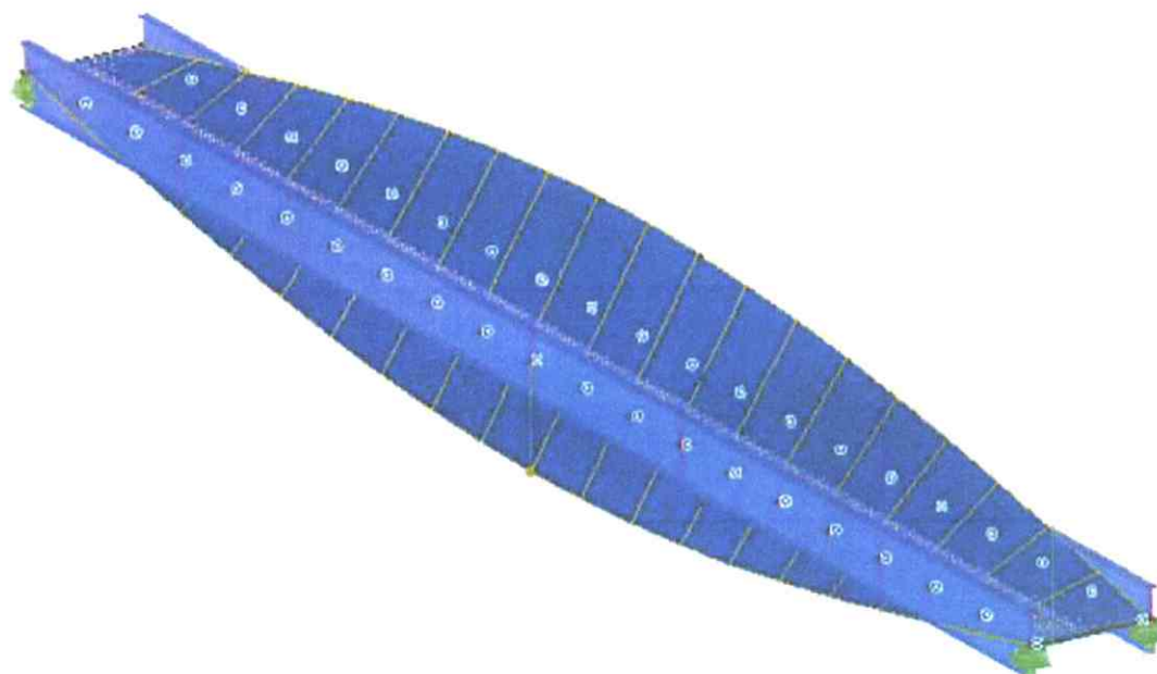
Obr. 4.5 – II. vlastní tvar nezatížené konstrukce, ztužené monolitickou spřaženou betonovou deskou, f_2 = 3,76 Hz.
