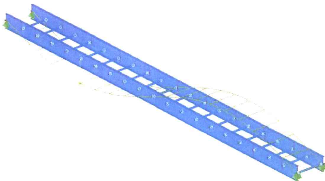
Obr. 4.2 – II. vlastní tvar nezátížené nevyztužené konstrukce, f_2 = 12,67 Hz.
