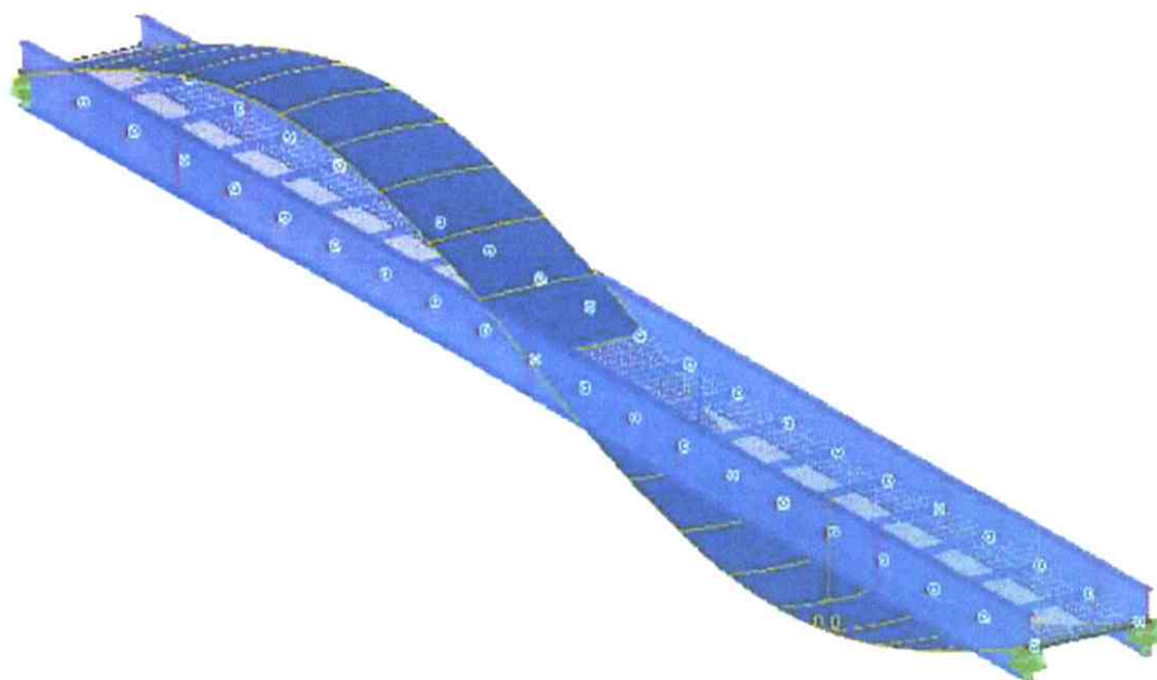
Obr. 4.6 – III. vlastní tvar nezatížené konstrukce, ztužené monolitickou spřaženou betonovou deskou, f_3 = 12,14 Hz.
