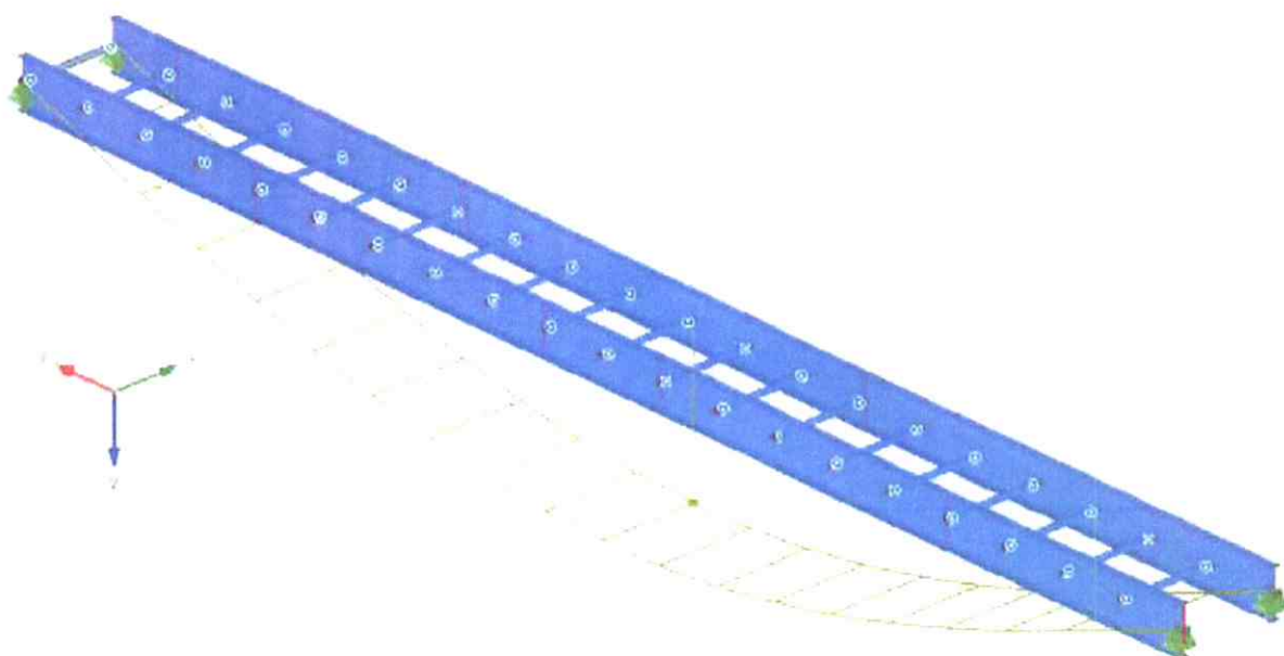
Obr. 4.1 – I. vlastní tvar nezatížené nevyztužené konstrukce, f_1 = 3,21 Hz.
