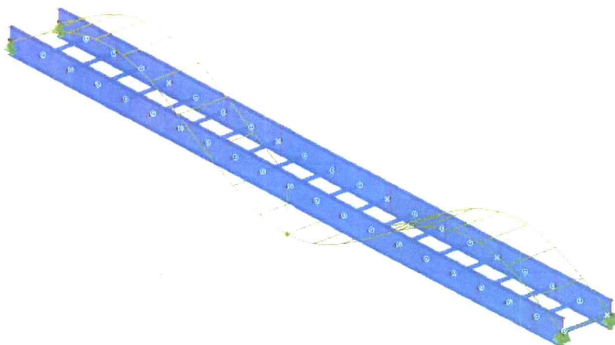
Obr. 4.3 – III. vlastní tvar nezátížené nevyztužené konstrukce, f_3 = 27,90 Hz.
