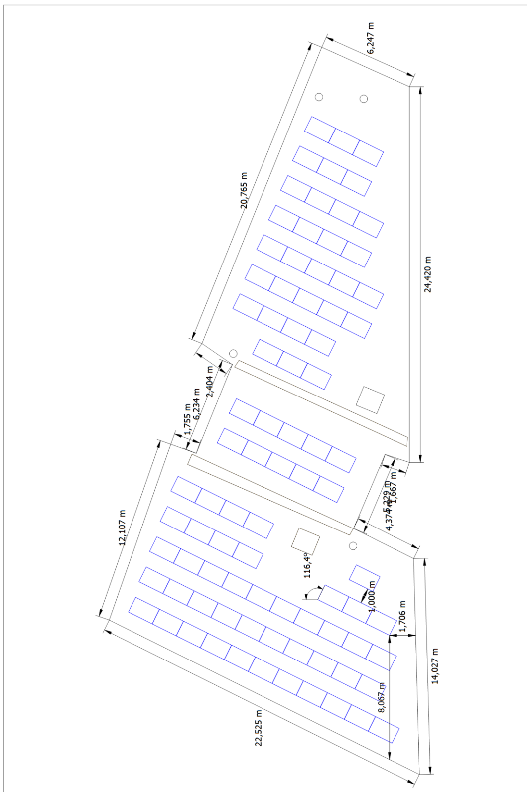
Obr.4 rozměrový výkres střechy
