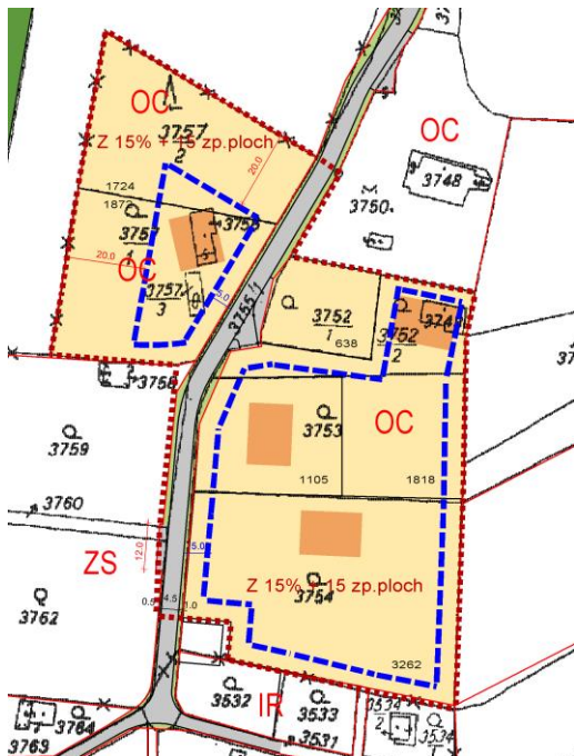
Výřez z hlavního výkresu RP Akátová
